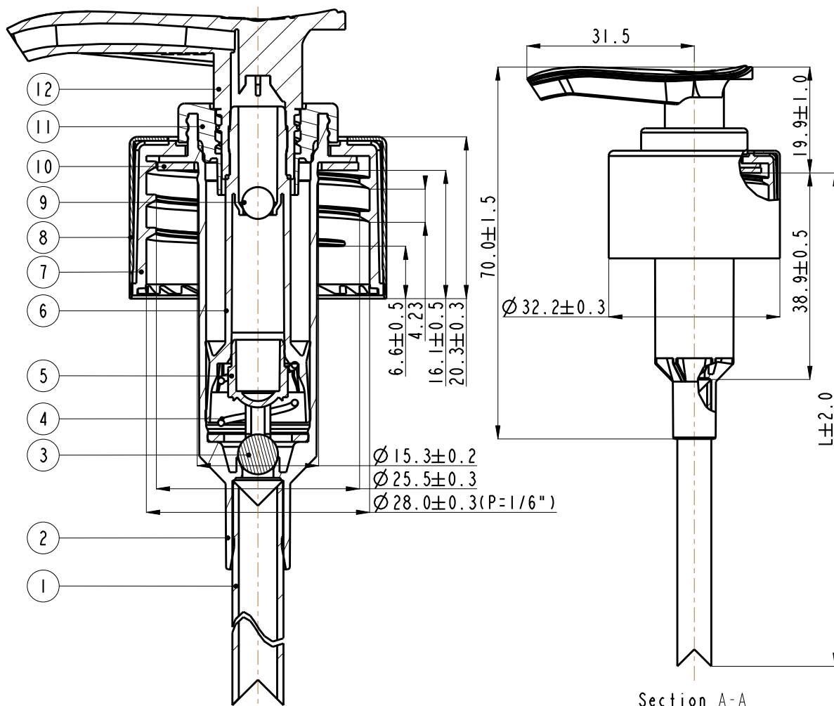
Section A-A
