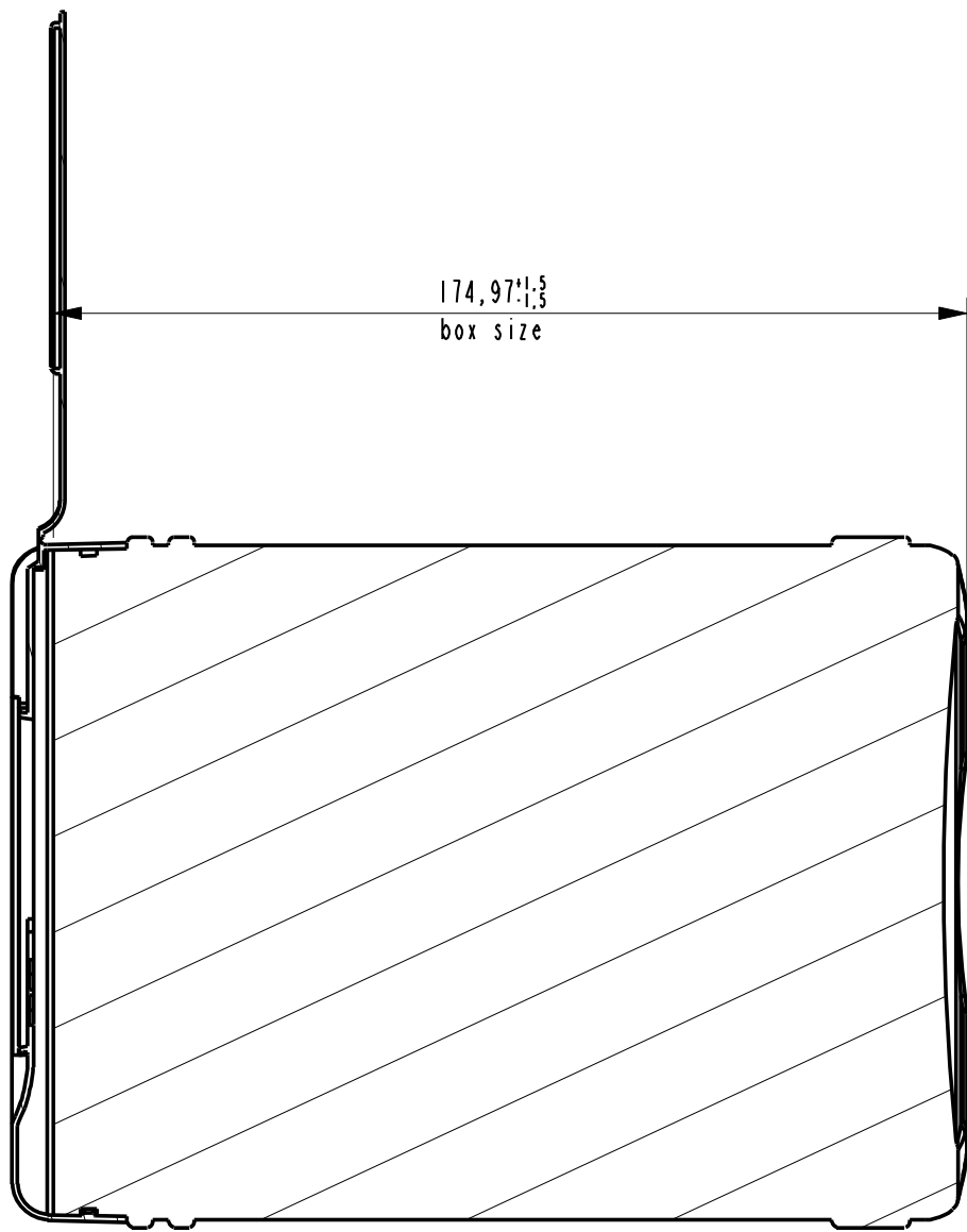
SECTION A-A
